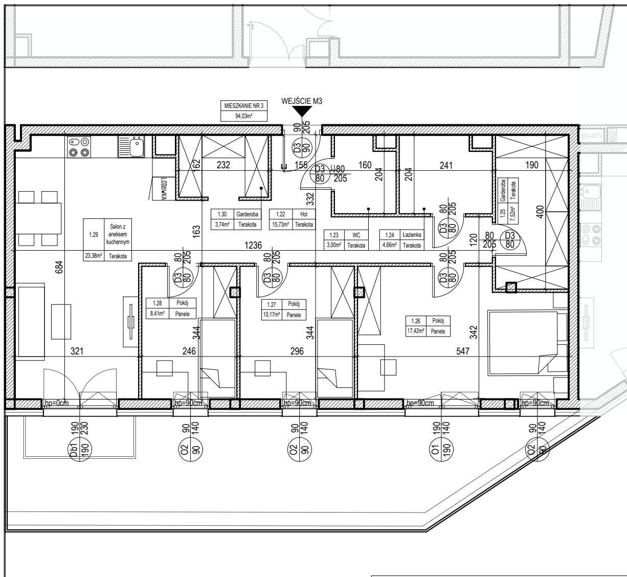
WYKAZ POWIERZCHNI - MIESZKANIE NR 3
